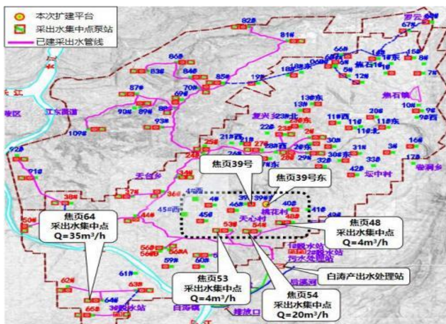
图 2.4-1 焦石坝区块中区产出水系统总体部署图
