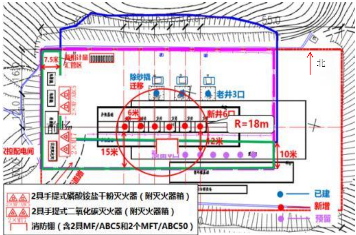
图 2.5-2 焦页 39 号东平台（新建）灭火器配置平面图
