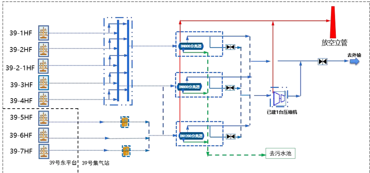
图 2.3-2 焦页 39 号东集气站工艺流程图
