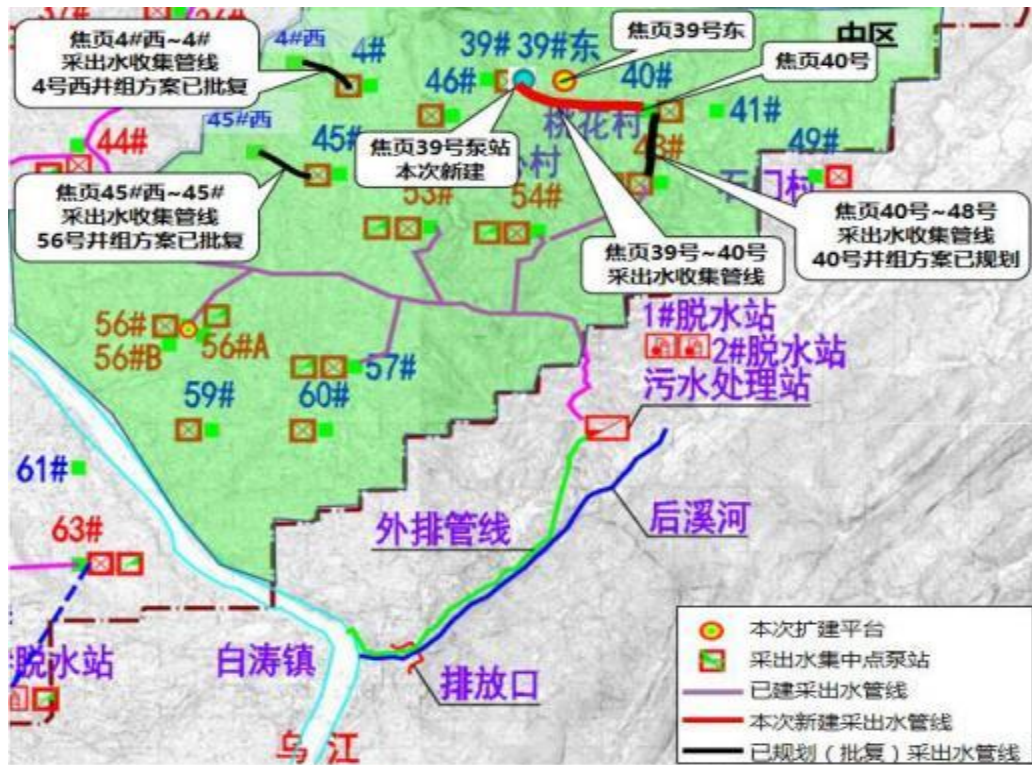
图 2.4-2 本方案新建采出水收集系统示意图
