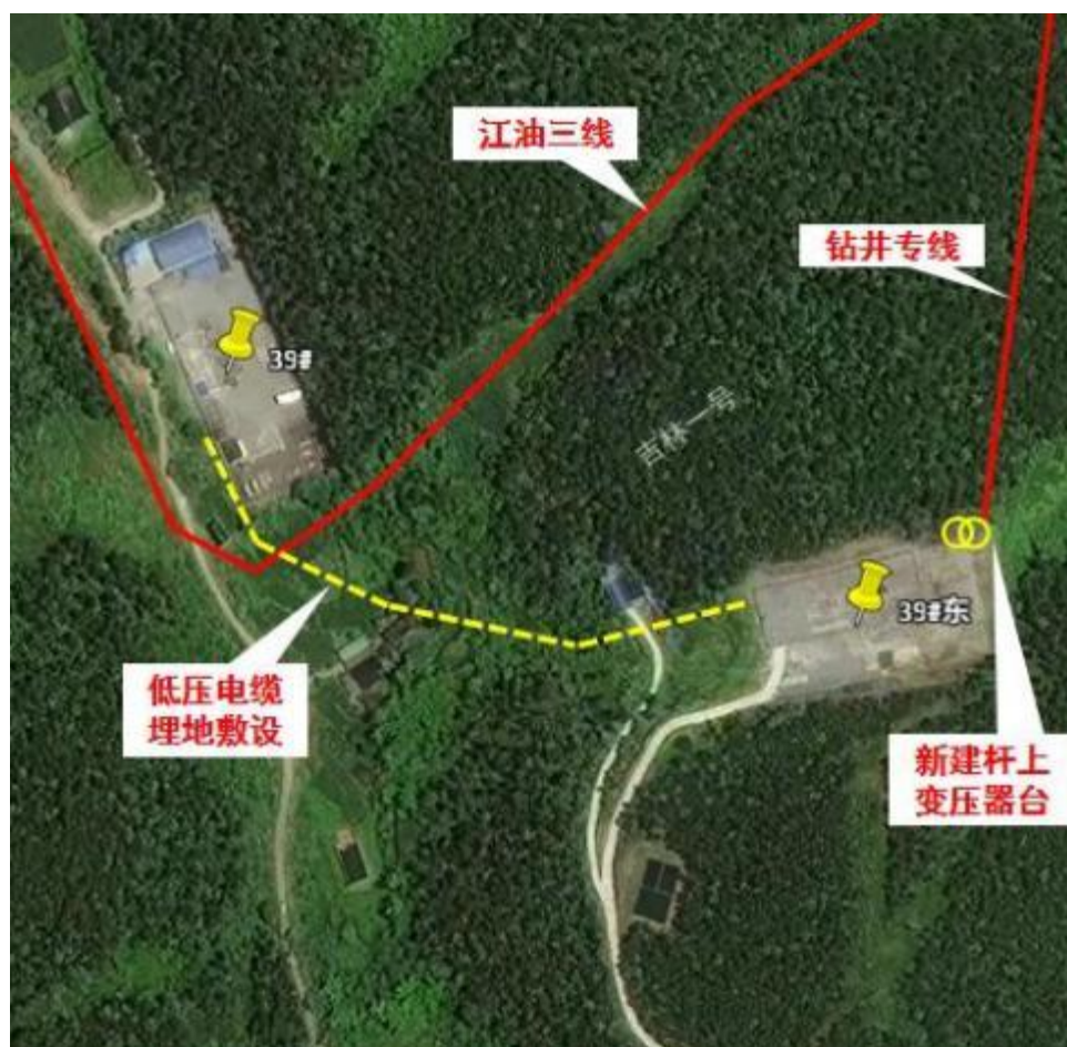
图 2.5-1 39 号东扩平台生产供电示意图
